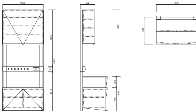
Beispiele für Konfigurationen: Grundmodul einfach, Modul mit Ober- und Unterschrank, Modul mit Tablaren und rechtsseitigem Korpus.
